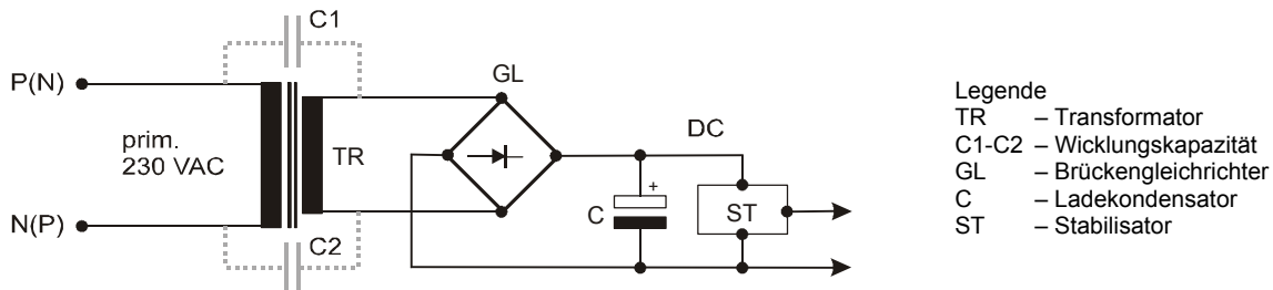
Abbildung 3: Typische Gleichrichterschaltung
