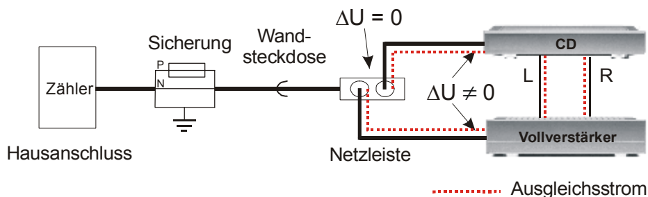
Abbildung 2: Entstehung von Differenzspannungen in den letzten 1,5m
